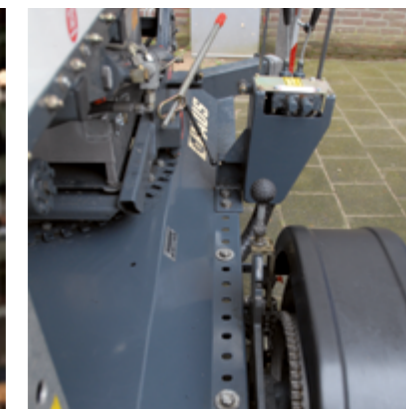
Radantrieb
